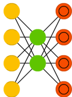
Auto-encoder
